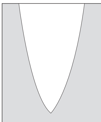
Balligschliff - richtig
